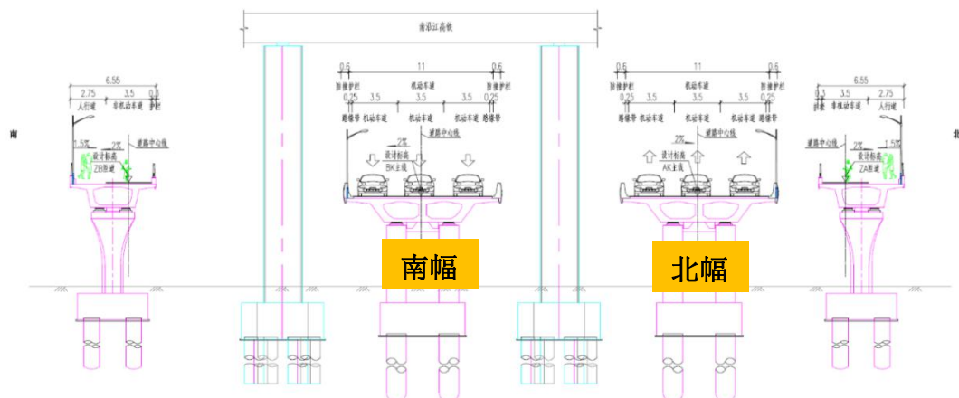
图 5 秦淮河西侧站前路主线含人非匝道段标准横断面图
