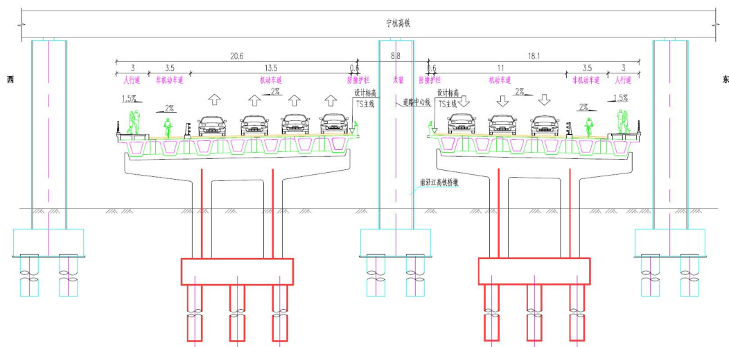
图 9 土山路主线高架桥段标准横断面图
