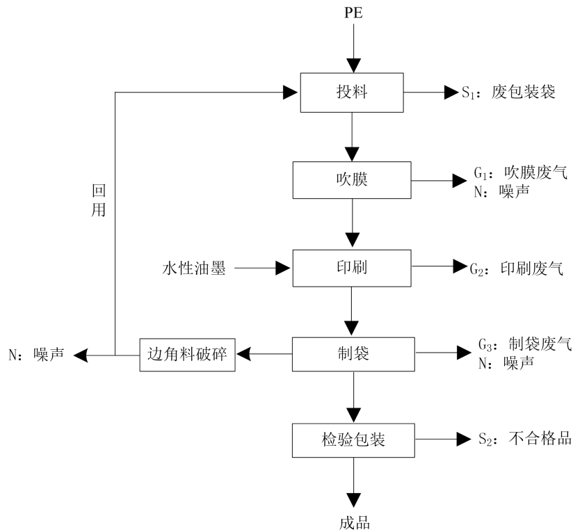
图 2-2 塑料袋生产工艺流程图
