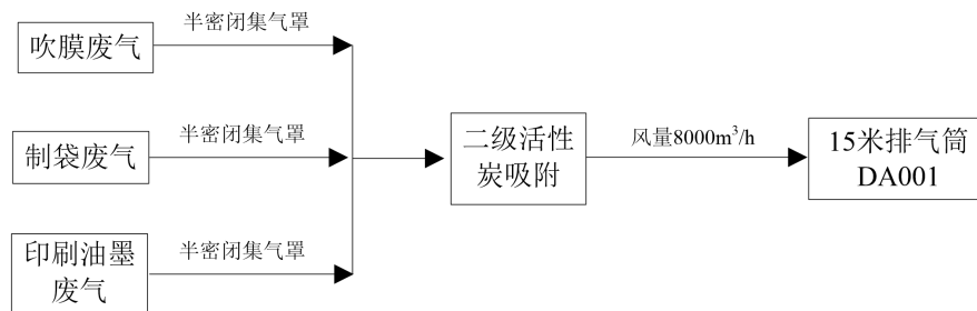
图4-1 废气治理及排放措施
